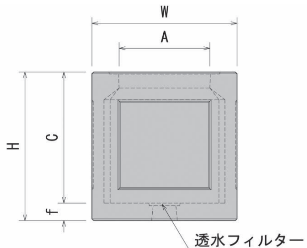
側面図
