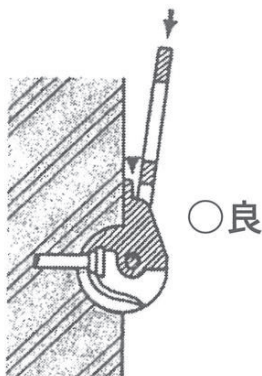
直角方向に吊る場合の作動状況
