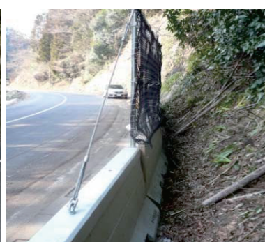
施工後：落石混じり土砂を捕捉
