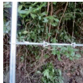
横ロープとPSターンバックルの接続
